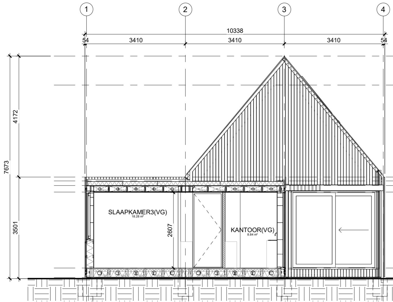
DOORSNEDE Y-1
