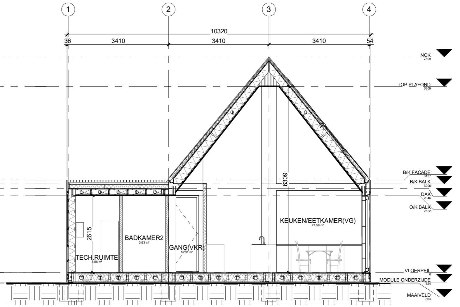
DOORSNEDE Y-2
